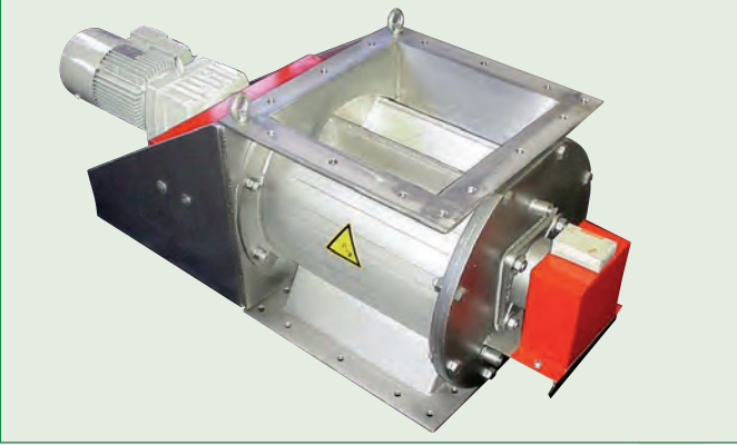
स्टेनलेस स्टील से बना रोटरी वॉल्व
