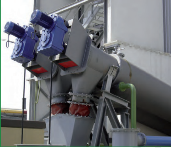
मट्टी के लिए पाइप कूलिंग स्कूर
