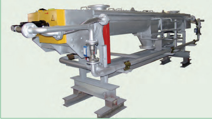
ट्रफ कूलिंग स्कू कन्वेयर में शामिल हैं वाटर पाइपिंग
