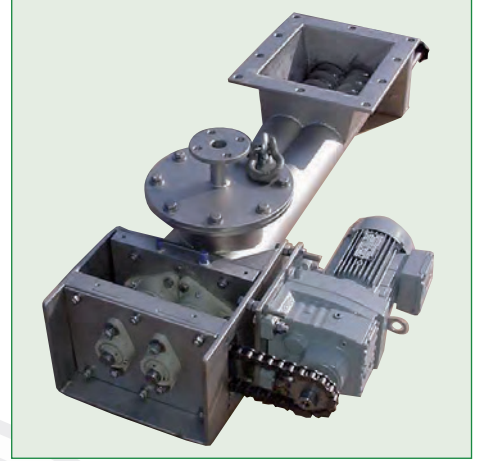
स्टेनलेस स्टील में डबल पाइप डोजिंग स्कू
