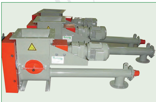
पृथक स्टरिंगि इकाई वाला फाइन डोजिंग स्कू
